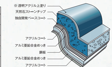
断面構成図
